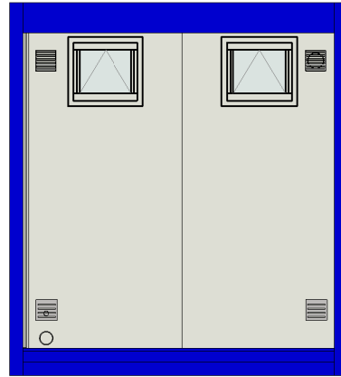
ARRIERE Ech : 1 : 50
